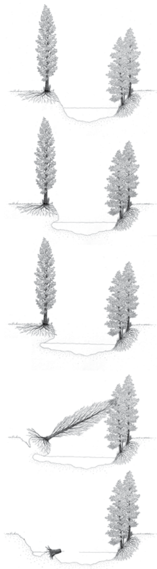
Le peuplier hybride en bord de rivière peut provoquer l'érosion des berges et la formation d'embâcles
