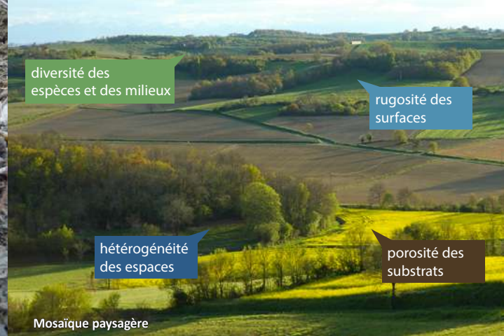
Une terre profonde et poreuse, riche en matière organique (humus) et vivante (activité biologique) dispose d'une bonne capacité d'absorption et de rétention
